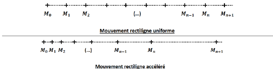
Figure 6.4 – Exemples de chronophotographies de mouvements rectilignes.
