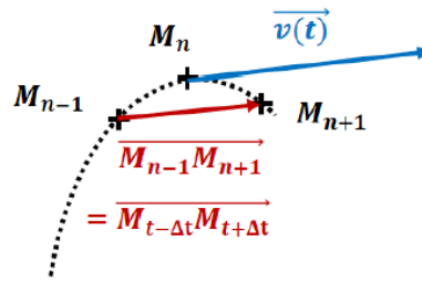
Figure 6.2 – Schéma représentant le vecteur vitesse instantanée moyen entre ses deux plus proches voisins
