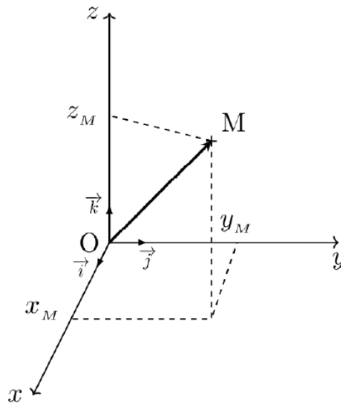
Figure 6.1 – Vecteur position d'un point M dans un repère orthonormé
