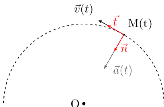
Figure 6.5 – Schéma représentant le repère de Frenet dans le cas d'une trajectoire circulaire
